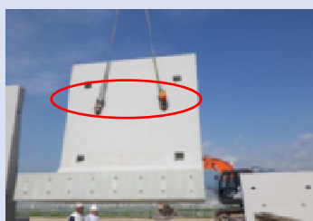
玉掛警報器による安全対策
